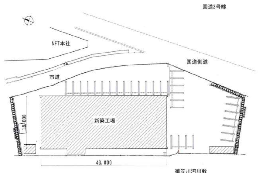
配置図
